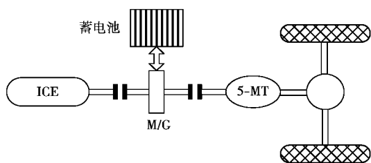
图 1 中度混合动力汽车结构简图
