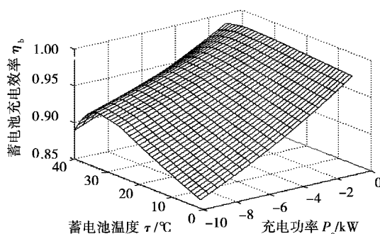
(a)SOC 为 0.5 时的蓄电池充电效率
