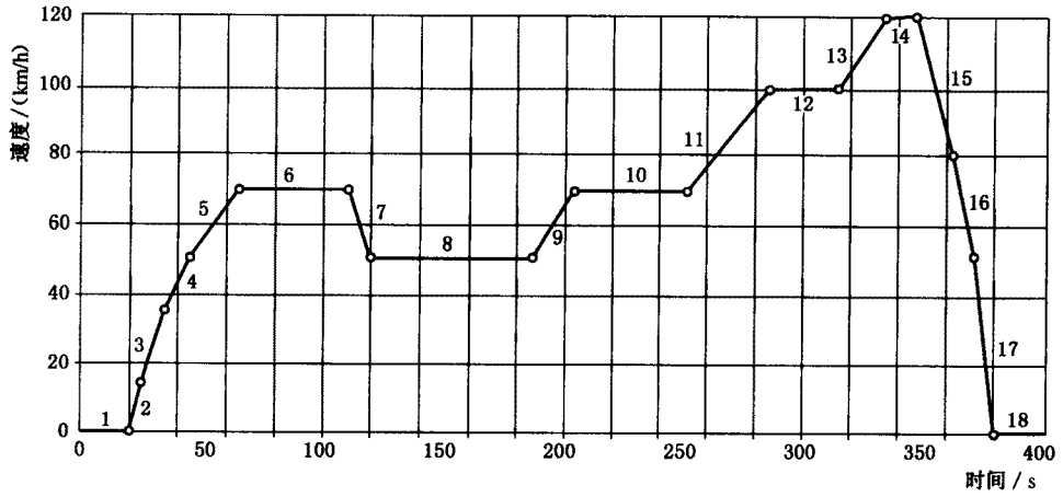
图 A.3 市郊循环
