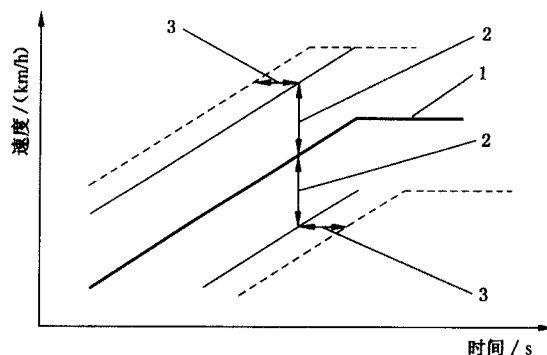
图中：1——基准曲线； 2——速度公差，单位为千米每小时(km/h)； 3——时间公差，单位为秒(s)
